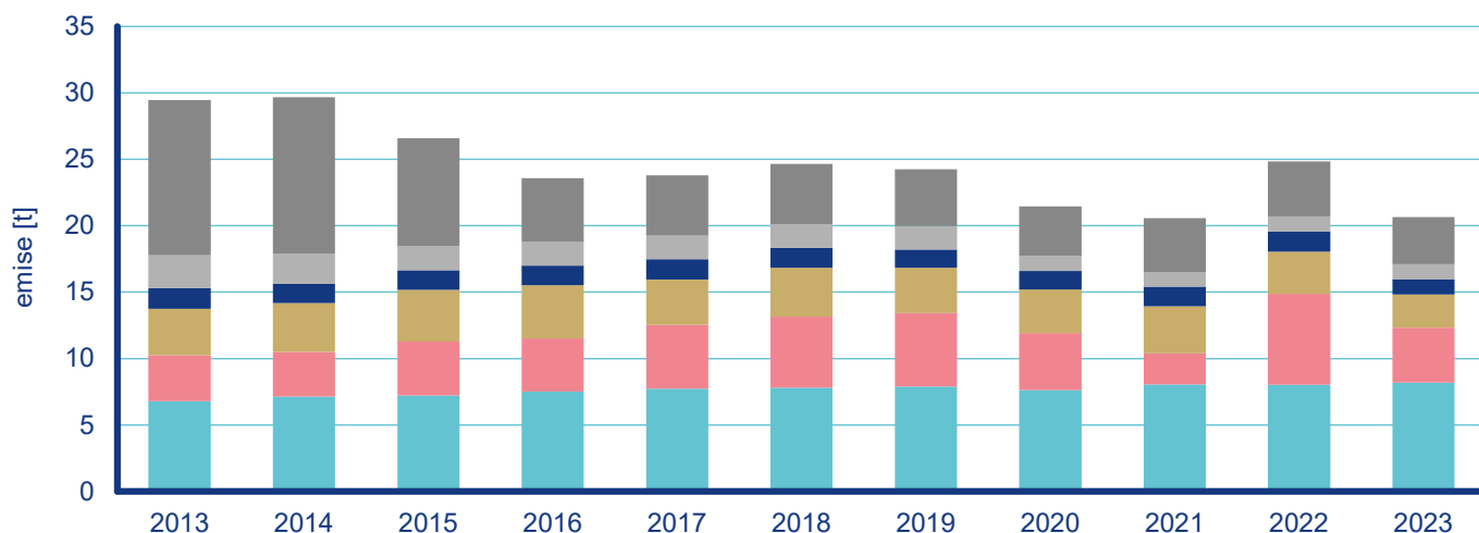
Obr. IV.6.21 Vývoj celkových emisí olova, 2013–2023
