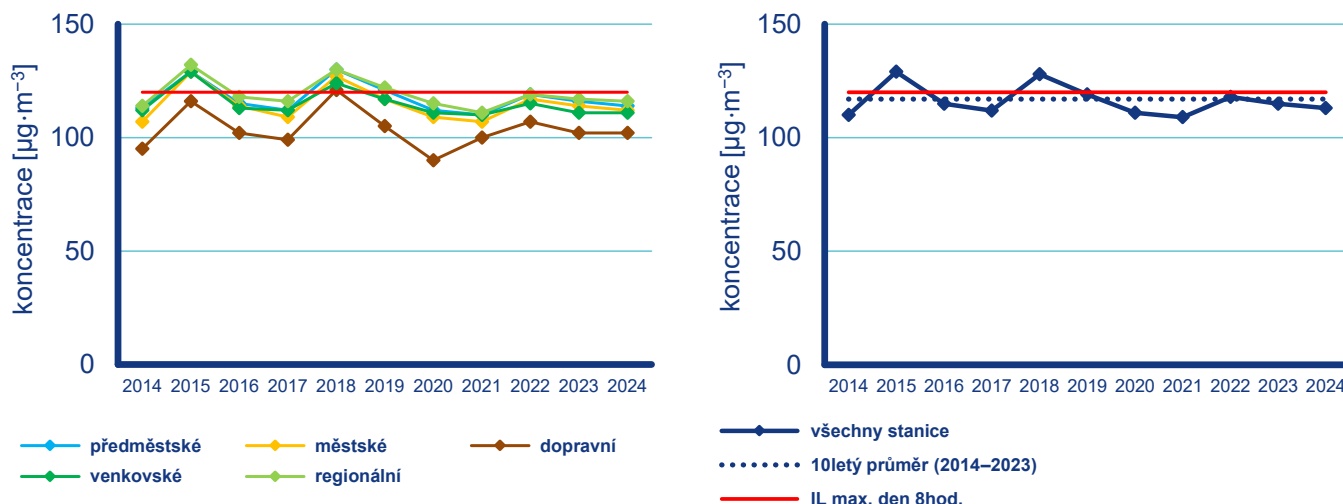
Obr. IV.4.10 Koncentrace přízemního \text{O}_3 (26. nejvyšší max. denní 8hod. klouzavý průměr), 2014–2024
