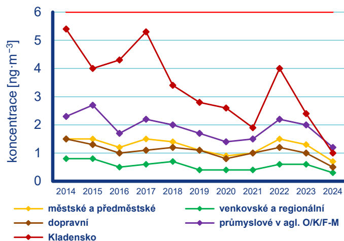
Obr. IV.6.10 Roční průměrné koncentrace arsenu, 2014–2024
