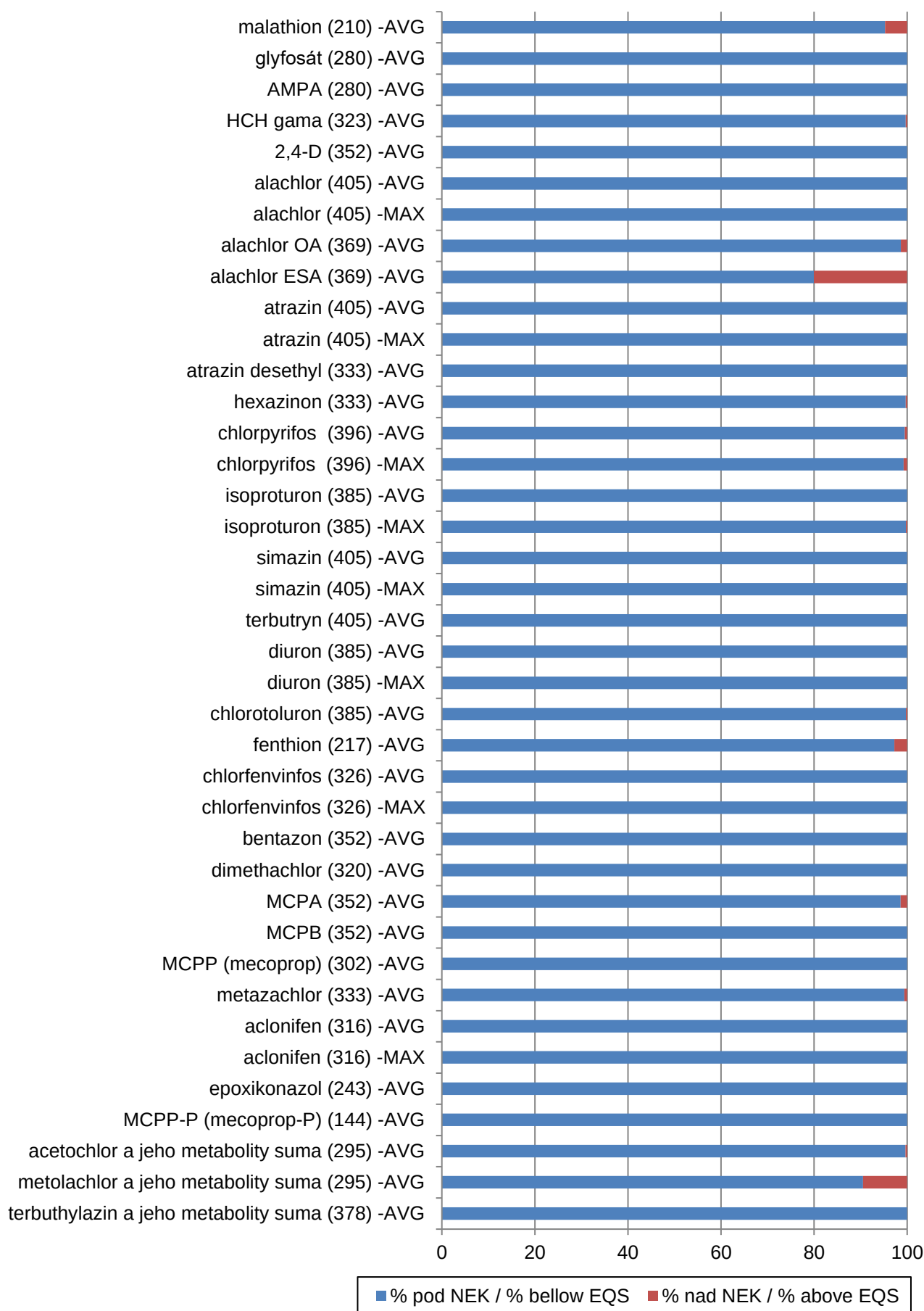
Obr. III.16E Překročení NEK u pesticidů dle Nařízení vlády č. 401/2015 Sb. v roce 2018.
