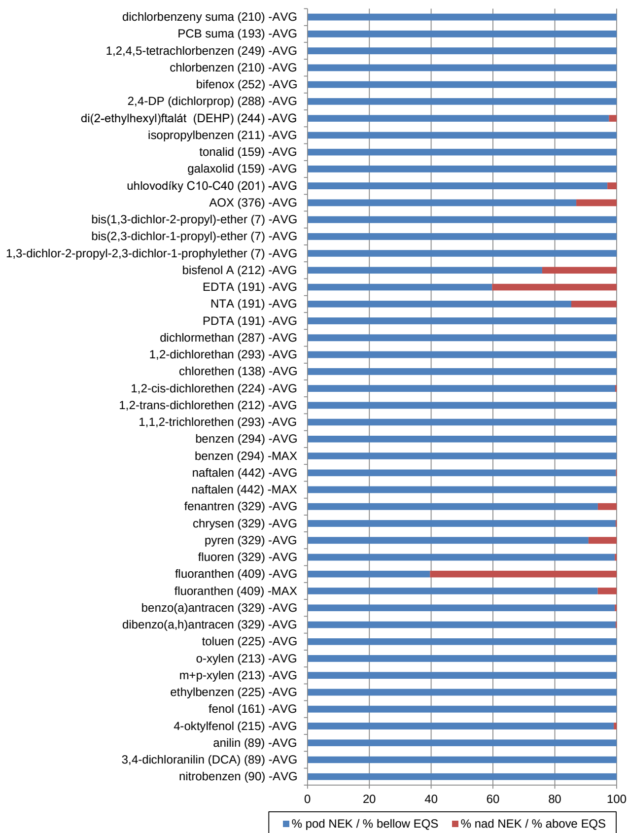
Obr. III.17E Překročení NEK u ostatních látek dle Nařízení vlády č. 401/2015 Sb. v roce 2018.
