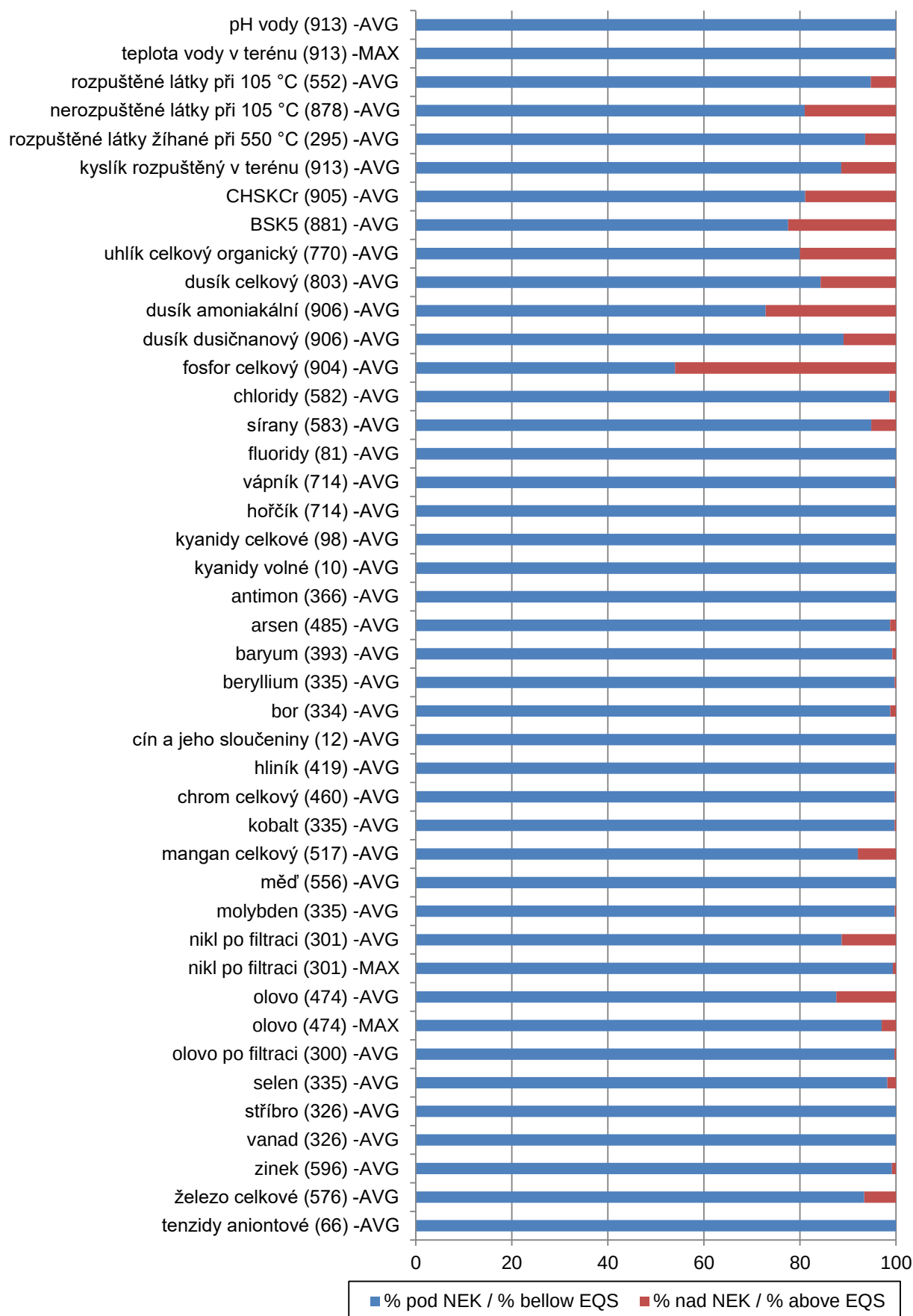
Obr. III.14 Překročení NEK u všeobecných ukazatelů dle Nařízení vlády č. 401/2015 Sb. v roce 2018. Fig. III.14 General determinands above EQS of Government Order No. 401/2015 Coll. in 2018.
