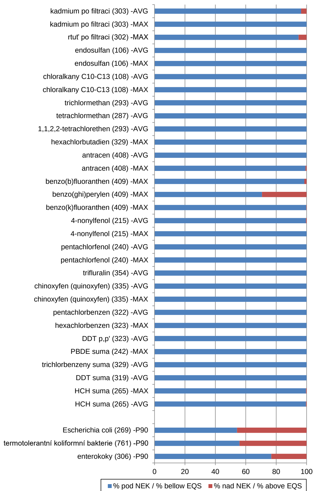
Obr. III.15E Překročení NEK u prioritních látek a mikrobiologických ukazatelů dle Nařízení vlády č. 401/2015 Sb. v roce 2018. Fig. III.15E Priority and microbiological determinands above EQS of Government Order No. 401/2015 Coll. in 2018.
