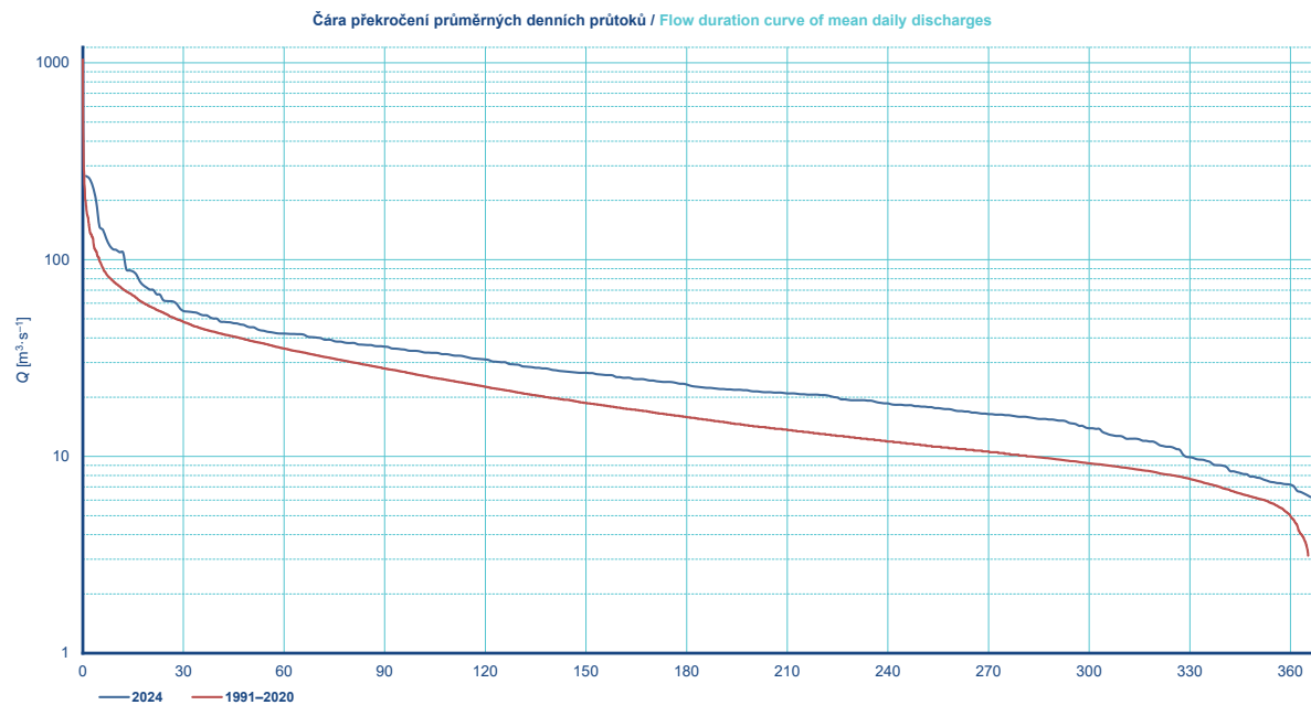
Obr. I.2.6 Hydrologické údaje z vodoměrné stanice Písek za rok 2024. Fig. I.2.6 Hydrological data from the Písek water gauging station in 2024.
