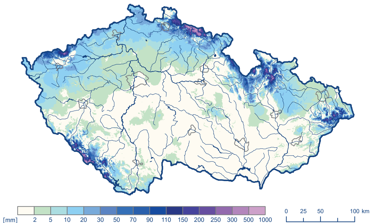
Mapa I.1.4 Největší zásoba vody ve sněhové pokrývce na území České republiky v roce 2024 (22. 1. 2024, 0,781 mld. m 3 , odtoková výška 9,9 mm) .
