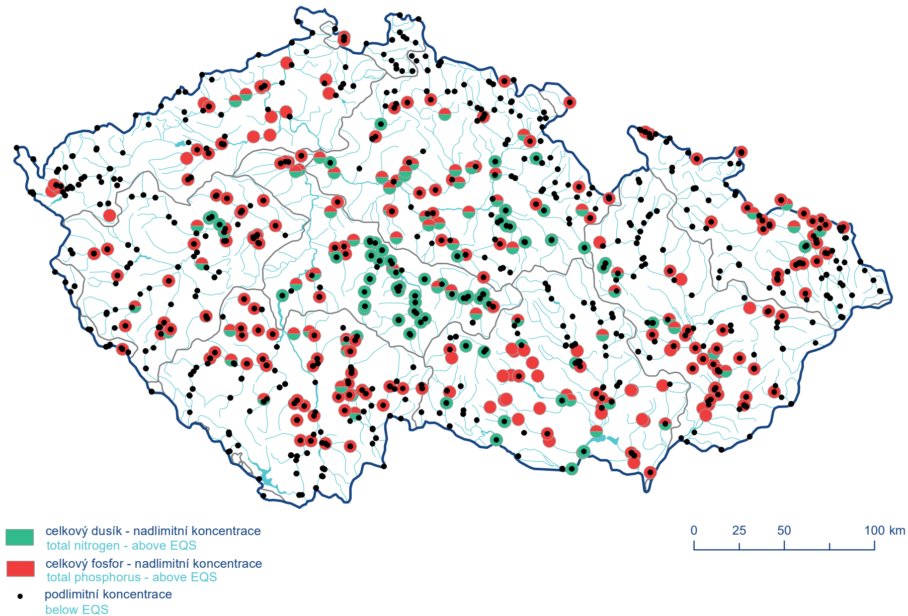
Mapa III.1.11 Koncentrace celkového dusíku a celkového fosforu v povrchových vodách v porovnání s NEK dle NV č. 401/2015 Sb. v roce 2024 Map III.1.11 Concentrations of total nitrogen and total phosphorus in surface water compared with the EQS of Government Order No. 401/2015 Coll. in 2024.
