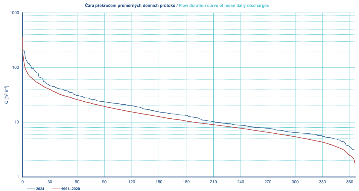
Obr. I.2.1 Hydrologické údaje z vodoměrné stanice Týniště nad Orlicí za rok 2024. Fig. I.2.1 Hydrological data from the Týniště nad Orlicí water gauging station in 2024.
