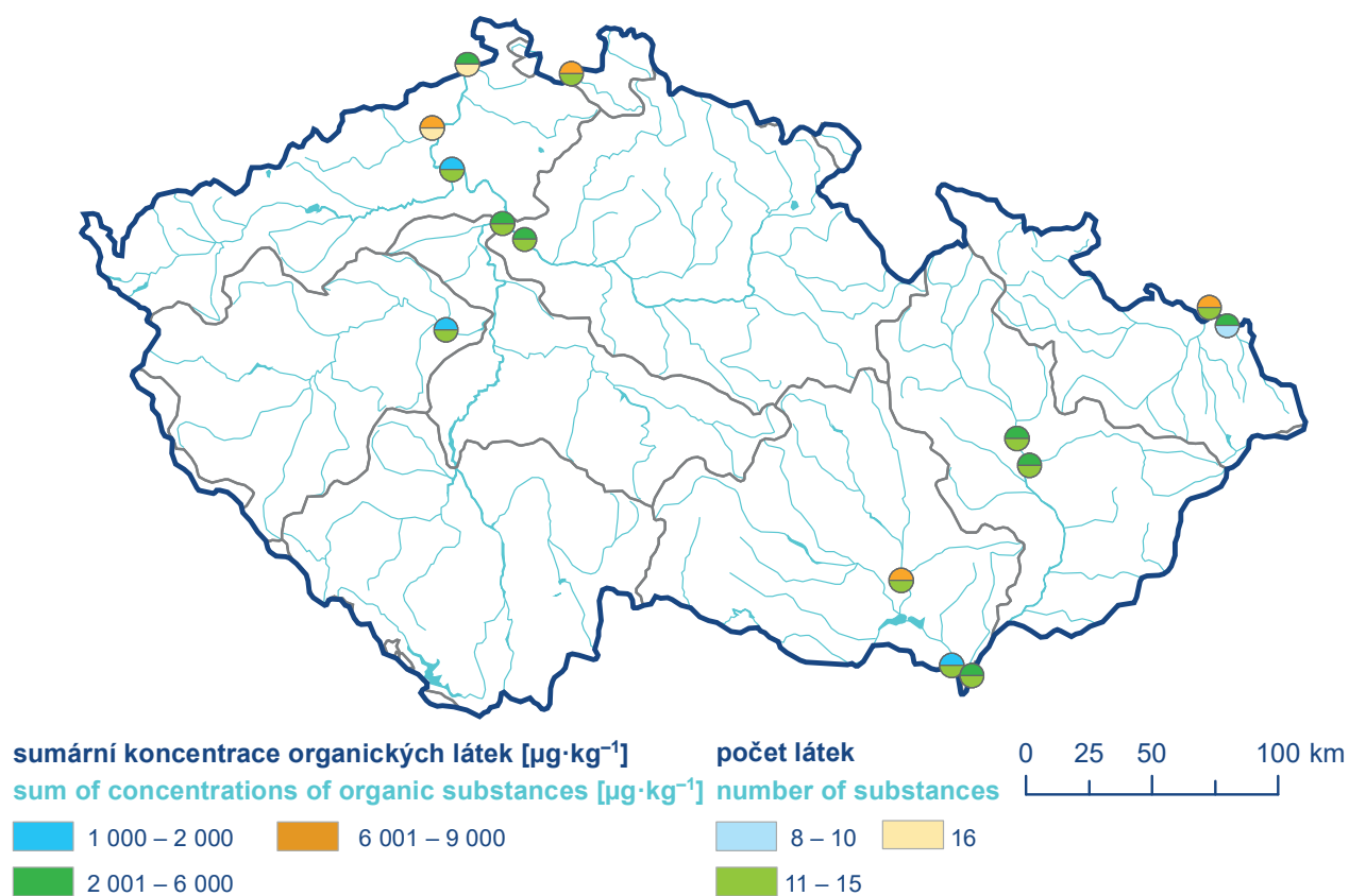
Mapa III.3.5 Sumy průměrných koncentrací prioritních látek Směrnice Evropského Parlamentu a Rady 2013/39/EU v sedimentovatelných plaveninách.
