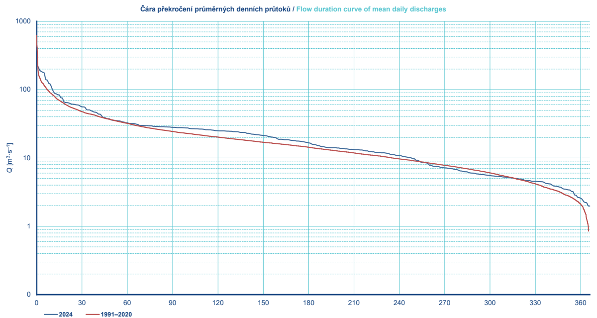
Obr. I.2.5 Hydrologické údaje z vodoměrné stanice Bechyně za rok 2024. Fig. I.2.5 Hydrological data from the Bechyně water gauging station in 2024.
