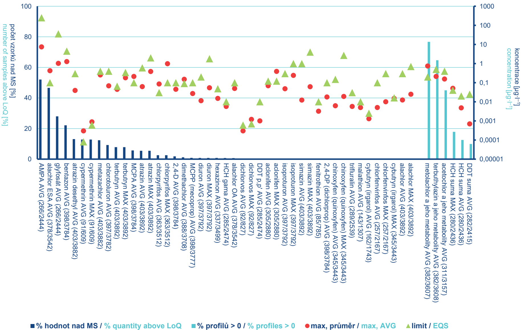
Obr. III.1.6 Procenta překročení MS, maxima a NEK v povrchových vodách pro pesticidy dle NV č. 401/2015 Sb. v roce 2024 (na ose X v závorce: počet sledovaných profilů / počet vzorků za rok). Fig. III.1.6 Percentage above LoQ, maximum and EQS in surface water for pesticides according to Government Order No. 401/2015 Coll. in 2024 (on the X axis in parentheses: number of observed profiles / number of samples per year).
