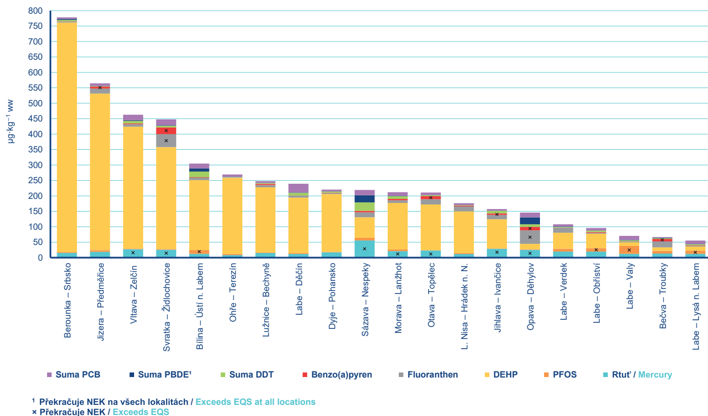
Obr. III.5.3 Koncentrace nebezpečných látek v matici bentos.
