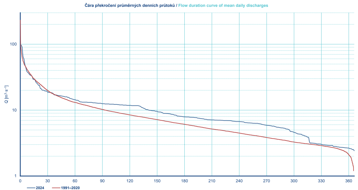
Obr. I.2.19 Hydrologické údaje z vodoměrné stanice Ivančice za rok 2024. Fig. I.2.19 Hydrological data from the Ivančice water gauging station in 2024.
