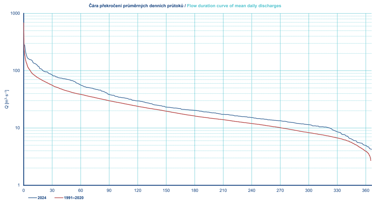
Obr. I.2.15 Hydrologické údaje z vodoměrné stanice Olomouc-Nové Sady za rok 2024. Fig. I.2.15 Hydrological data from the Olomouc-Nové Sady water gauging station in 2024.
